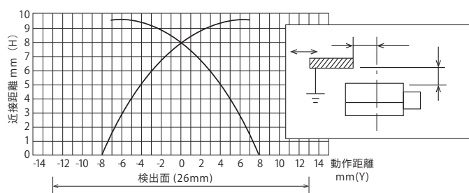
図1 従来センサ
