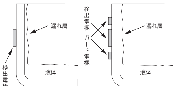
図1 従来センサ
